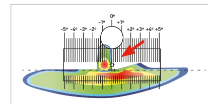
Beispiel Audi A8 mit Matrix-Beam-Fernlichtassistent Die vertikale Hell-Dunkel-Grenze lässt sich direkt auf der Skala ablesen. Die linke Grafik zeigt die korrekte Position an der Nulllinie. Bei Abweichungen von dieser Position (rechte Grafik) muss der Korrekturwert (Abstand zur Nulllinie) über einen Diagnosetester an das Steuergerät übertragen werden (hier am Beispiel des linken Scheinwerfers).
